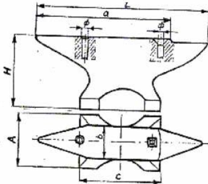
KOWADŁO DWUROŻNE RBKe
